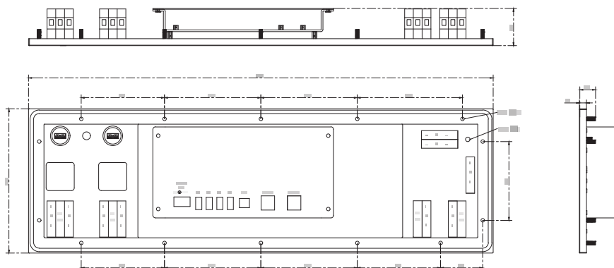
外形尺寸背视图
